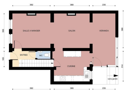
Rez-de-chaussée
