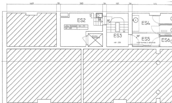
PLAN DE L'ENTRE-SOL 2
