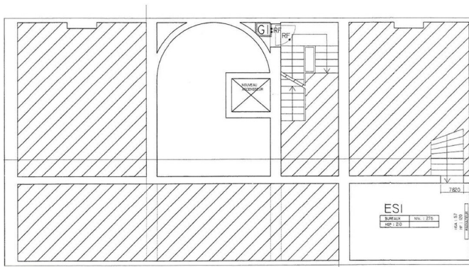
PLAN DE L'ENTRE-SOL
